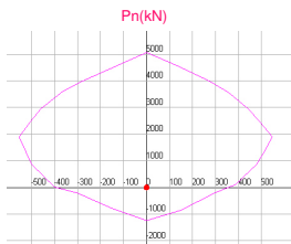
P-Mx-My Curve
